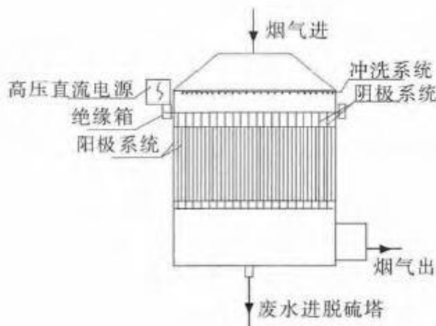
图 2 立式玻璃钢结构湿式除尘器的结构
