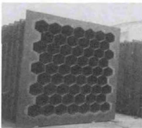
图 1 导电玻璃钢电除雾器结构
